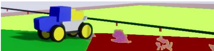
Abbildung 3 Simulation der variablen Ausbringungsmenge auf dem UNI-Sportplatz mit der Software Canoe (Vector) und einer Physik-Engine
