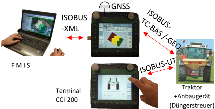
Abbildung 2 Herstellerübergreifende Kommunikation zwischen einem FMIS (links), einem Terminal (Mitte) und einem Traktor mit Anbaugerät (rechts)
