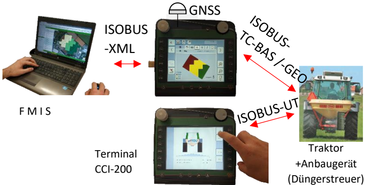
Abbildung 2 Herstellerübergreifende Kommunikation zwischen einem FMIS (links), einem Terminal (Mitte) und einem Traktor mit Anbaugerät (rechts)
